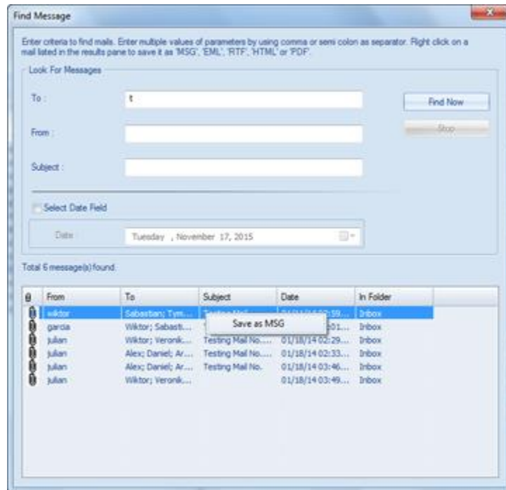
Find Message
